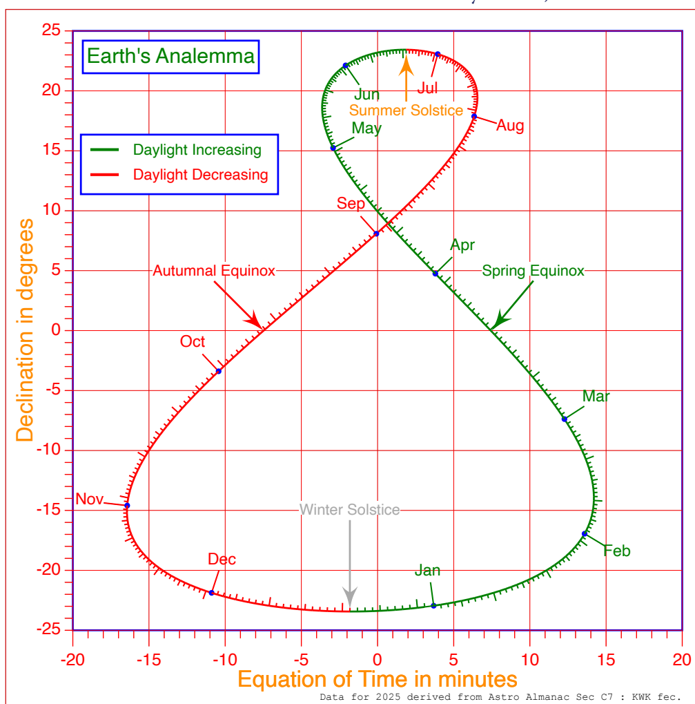
Fig 3 - The Analemma
