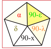
Fig. 12 : Right Ascension
