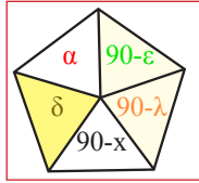
Fig. 11 : Declination
